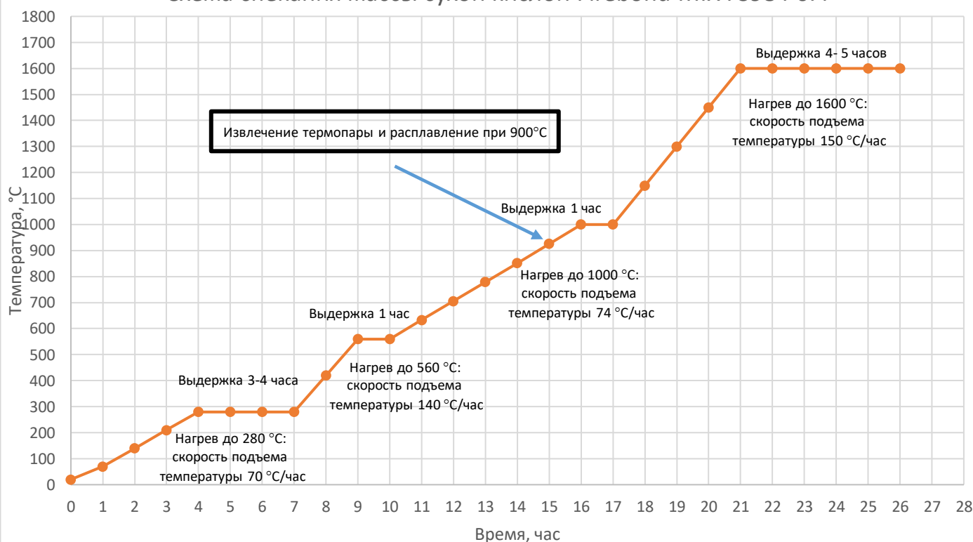
Схема спекания массы сухой кислой Firebond MIX FS984 0.4
