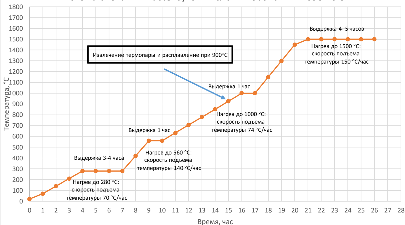
Схема спекания массы сухой кислой Firebond MIX FS982 0.8
