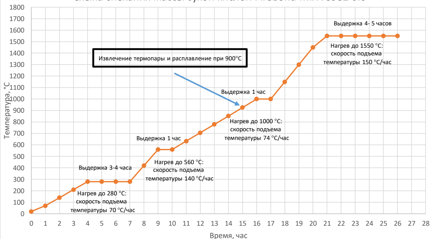
Схема спекания массы сухой кислой Firebond MIX FS982 0.6
