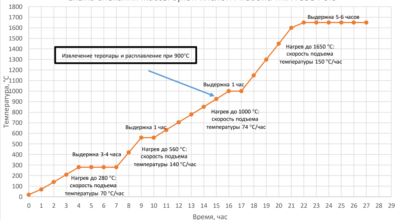
Схема спекания массы сухой кислой Firebond MIX FS984 0.0
