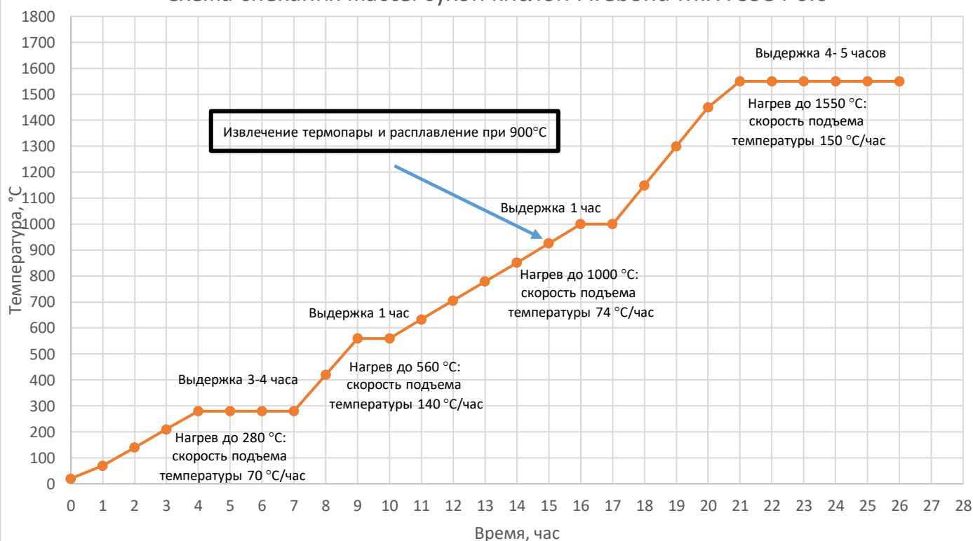
Схема спекания массы сухой кислой Firebond MIX FS984 0.6
